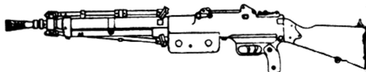
Fig. 1. — Côté gauche de l'arme.
